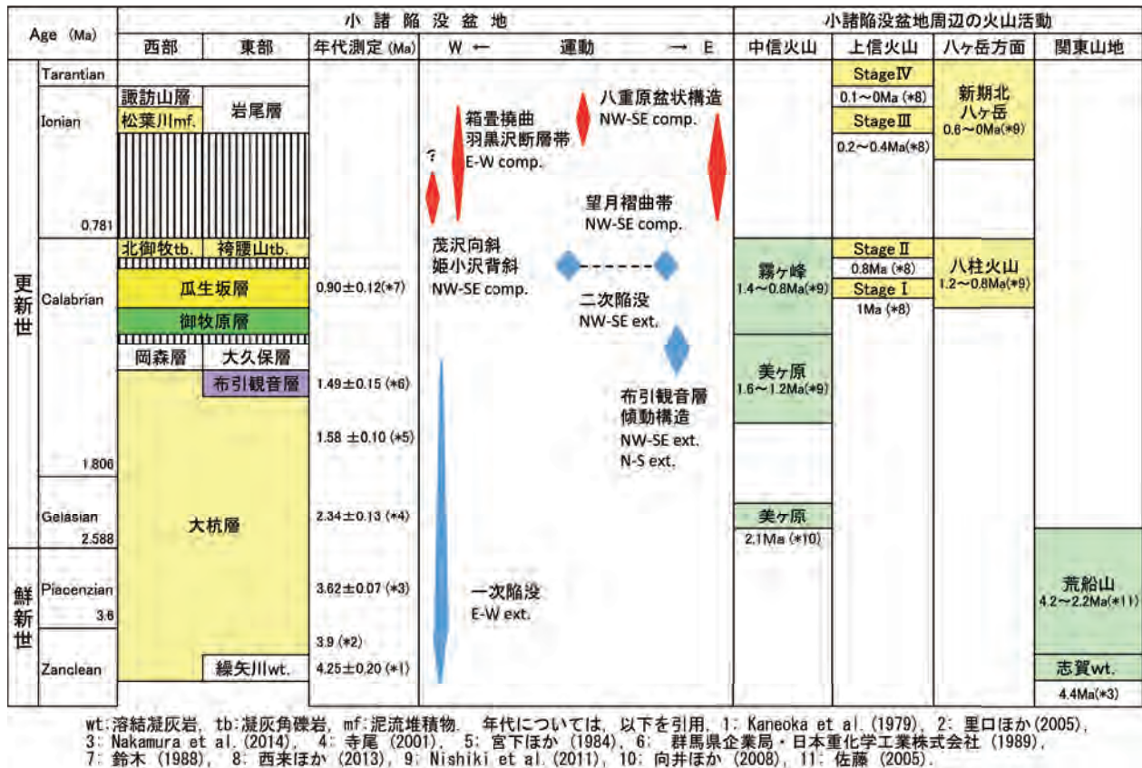
図7 小諸陥没盆地構成層の層序、地質構造形成および周辺の火山活動の時空配列。小諸層群最上部の八重原溶岩・氷溶岩は省略。図中央の運動の列内での青は張力場 (ext.), 赤は圧縮場 (comp.) での変形を示す。
