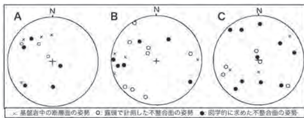
図8 調査域西縁部での基盤と小諸層群との不整合面および基盤中の固結した断層面の極のπ-ボールダイアグラム (シュミットネット下半球使用)。A~Cの位置は図6参照, Bは図9内の範囲を含む。
