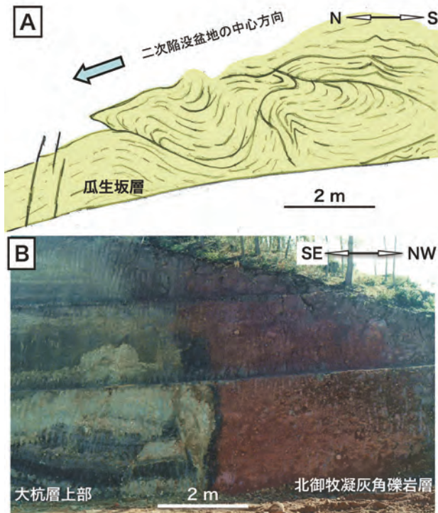
図14 二次陥没構造縁辺部の状況（位置は図6参照）。A：氷および鹿曲川陥没構造接合地付近での陥没盆地側に向かってスランプ褶曲した瓜生坂層の泥岩層，B：鹿曲川陥没盆地側に緩傾斜した大杭層上部と無層理の北御牧凝灰角礫岩層との高角アバット不整合関係。
