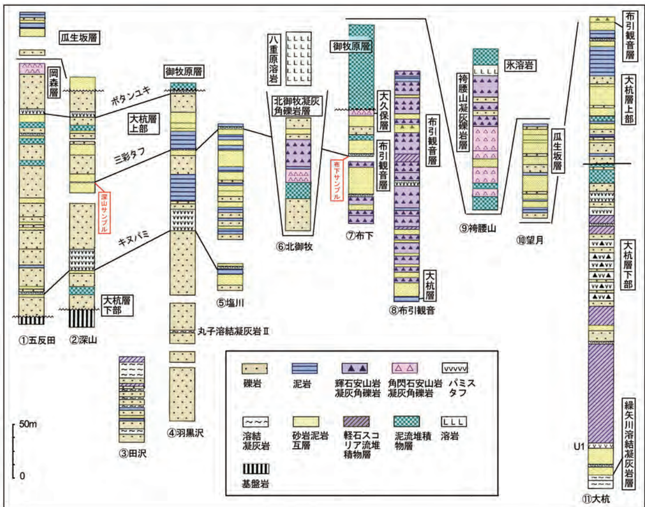
図5 八重原・御牧原盆地周辺の小諸層群の柱状図。作成位置は図3および本文参照。①～⑥は西部域，⑦～⑪は東部域。
