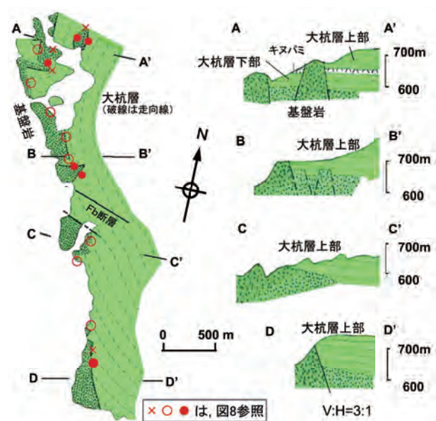
図9 一次陥没構造、図6のB地区周辺の地質図と断面図 (V:H=3:1)。断面図中の基盤岩と大杭層との接触面は、断層起源のアバット不整合面を含む。
